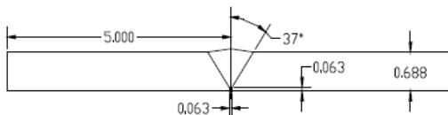
Disposição da Solda de Tubo 12" NPS
