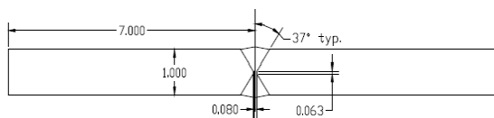
Disposição da Solda de Chapa 1"
